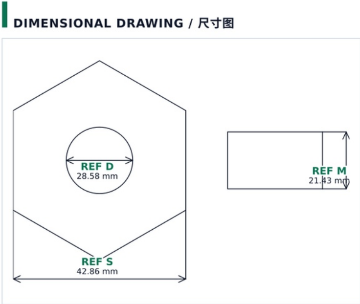
SCHEMATIC — NOT TO SCALE · ALL DIMENSIONS IN mm / 示意图—非按比例 · 尺寸单位: mm
